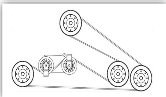
36" HGM
