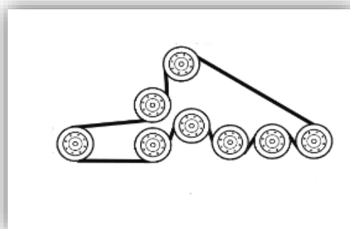
42" HGM
